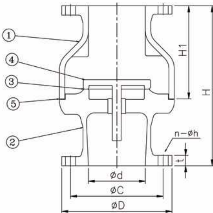
DIMENSION (Unit:mm)
